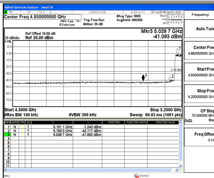
11AX40MIMO_Ant2_Low_5190
