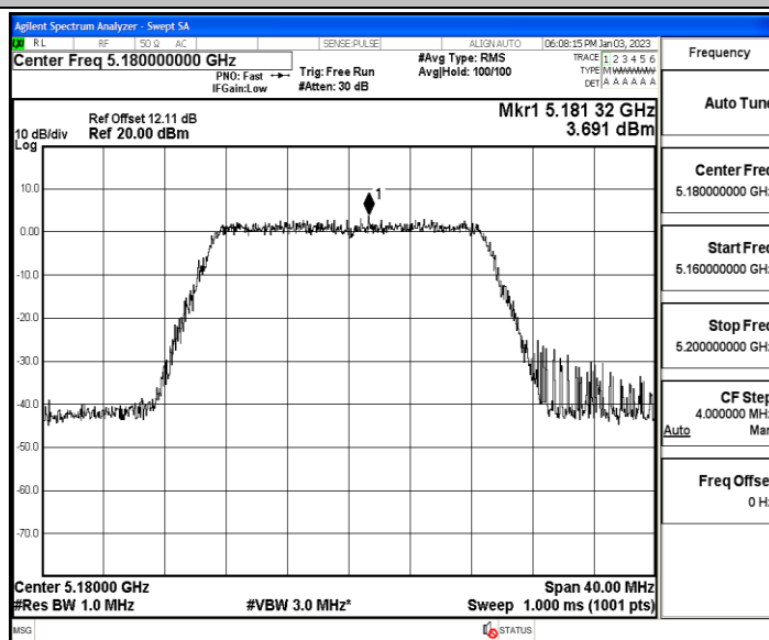
11AC20MIMO_Ant2_5180
