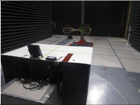
30-200 MHz
