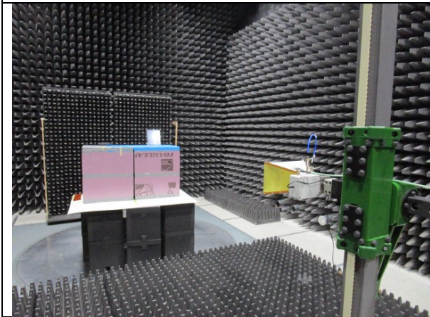
4-18GHz
