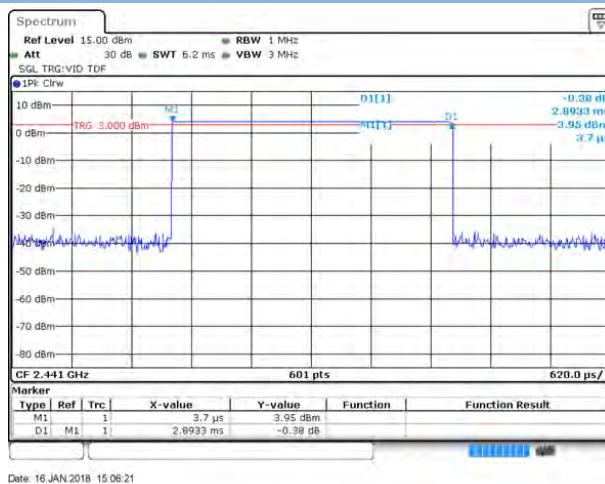
GFSK DH5
