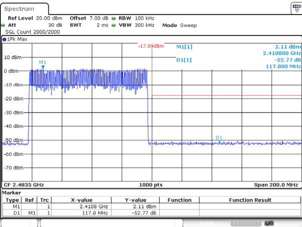
DH1_Hopping_Upper
