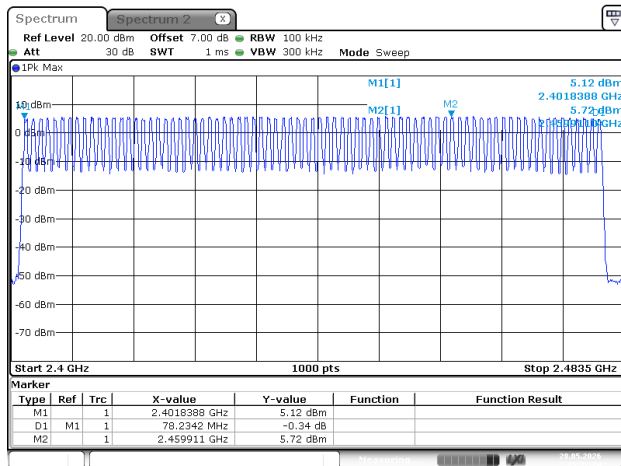
DH1_Hopping
