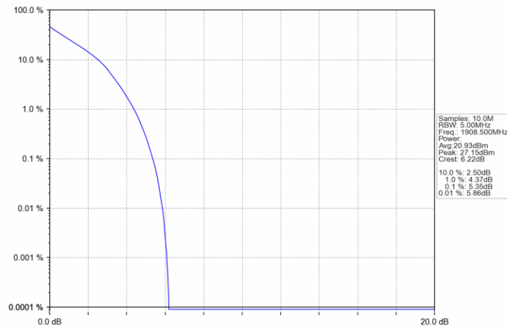
Band2_3MHz_QPSK_HCH_1908.5MHz_RB_15_0_NTNV
