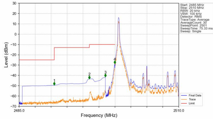
Band7_10MHz_QPSK_LCH_2505MHz_RB_1_0_NTNV
