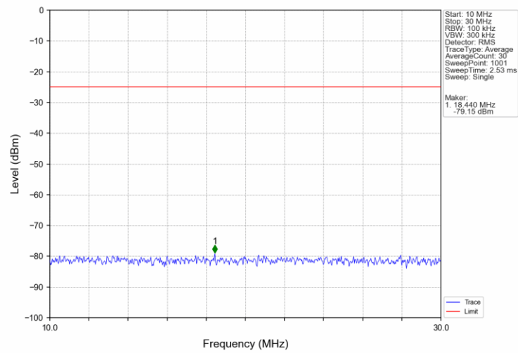
Band7_10MHz_QPSK_LCH_2505MHz_RB_1_0_NTNV
