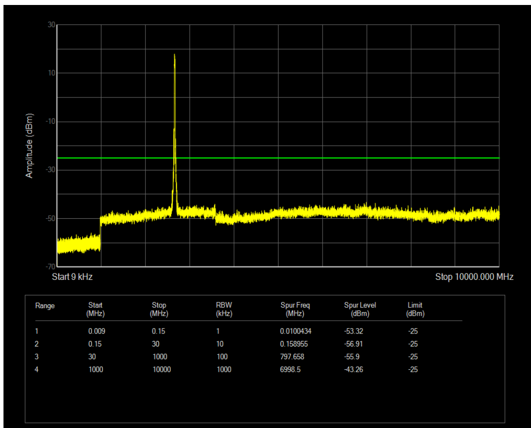
n41 SCS=30kHz CP_QPSK BW=20MHz Channel=535998 RB=1@0
