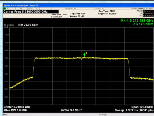
IEEE 802.11ax_Channel 42_80MHz_Antenna 0_RU&amp;Index SU
