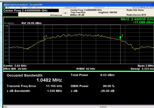
BLE 1M_Channel 19
