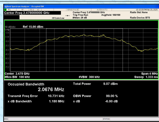
BLE 2M_Channel 38
