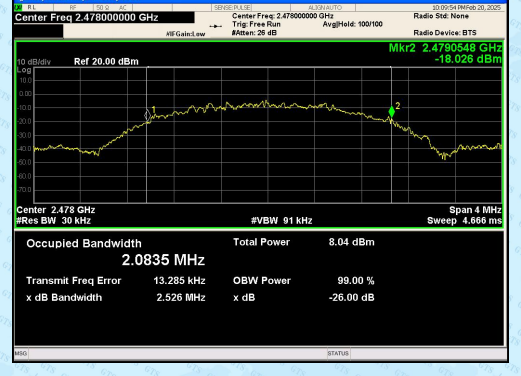
BLE 2M_Channel 38
