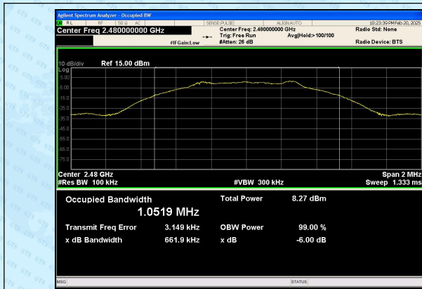
BLE 1M_Channel 39
