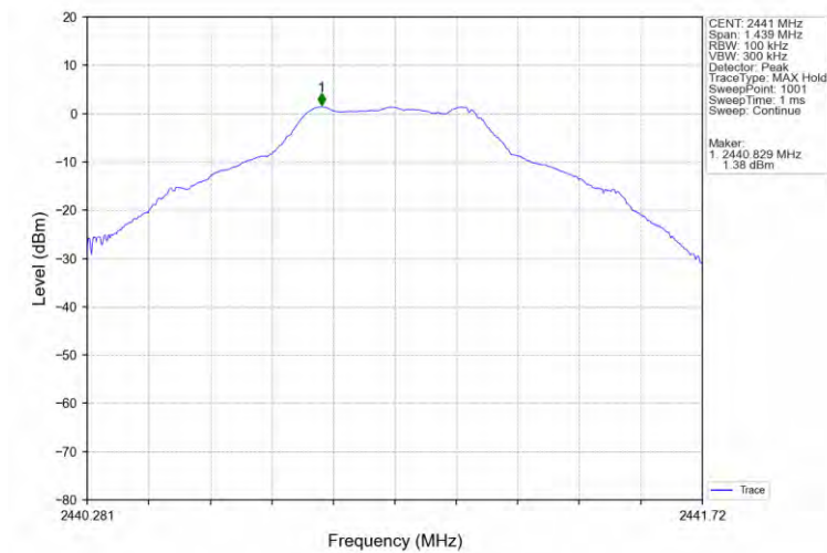
GFSK DH5 MCH 2441MHz Ant1 NTN
