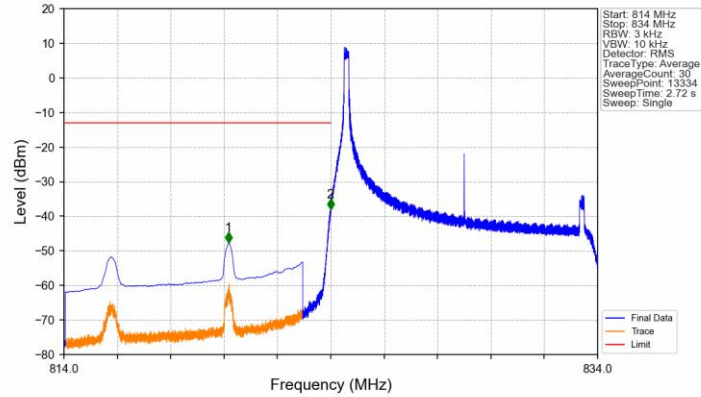
Band5_10MHz_QPSK_LCH_829MHz_RB_1_0_NTNV
