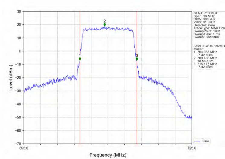
Band17_10MHz_QPSK_MCH_710MHz_RB_50_0_NTNV
