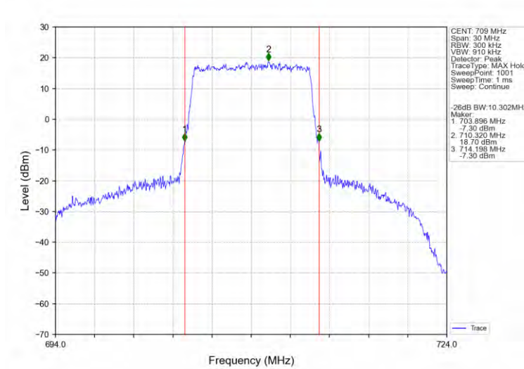
Band17_10MHz_QPSK_LCH_709MHz_RB_50_0_NTNV
