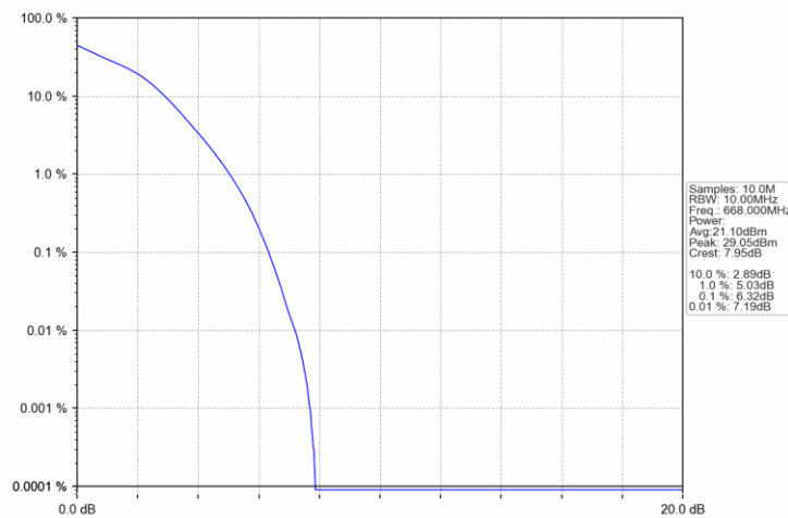
Band71_10MHz_16QAM_LCH_668MHz_RB_50_0_NTNV
