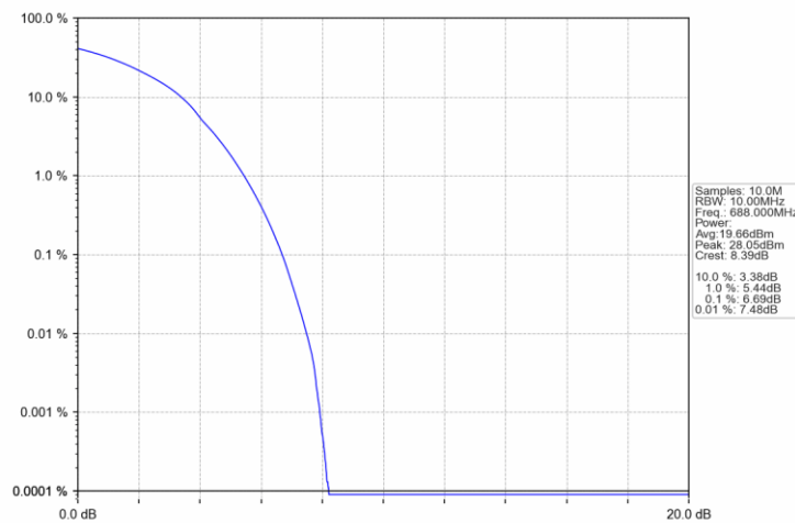
Band71_20MHz_16QAM_HCH_688MHz_RB_100_0_NTNV
