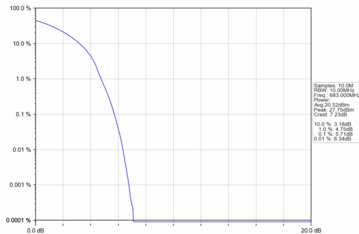
Band71_20MHz_QPSK_MCH_683MHz_RB_100_0_NTNV
