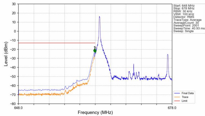
Band71_15MHz_QPSK_LCH_670.5MHz_RB_1_0_NTNV
