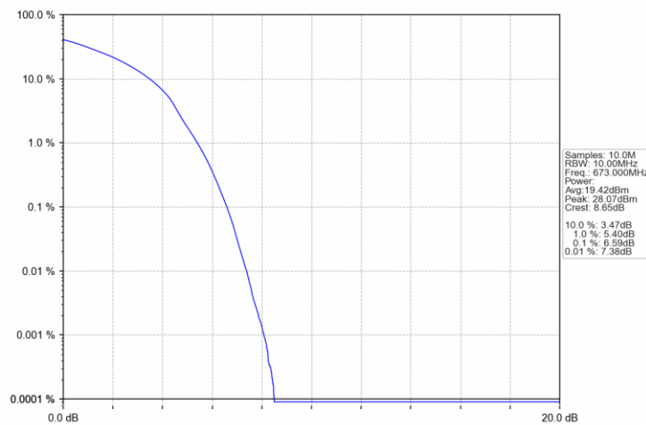
Band71_20MHz_16QAM_LCH_673MHz_RB_100_0_NTNV
