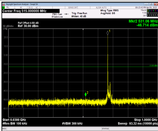
Band71-20MHz-QPSK-133372-1RB#0-Range1:30~1 000MHz
