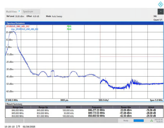
Band5_3MHz_16QAM_20635_1RB#0
