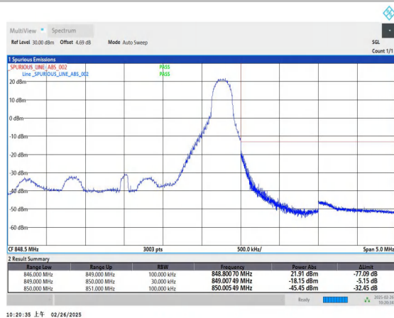
Band5_3MHz_16QAM_20635_1RB#14
