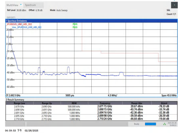
Band41_20MHz_QPSK_41490_1RB#0
