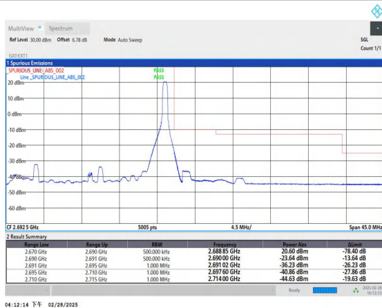
Band41_20MHz_QPSK_41490_1RB#99
