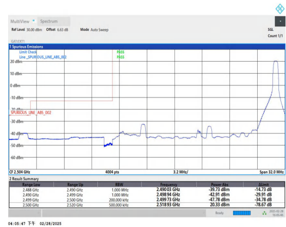
Band41_20MHz_QPSK_39790_1RB#99
