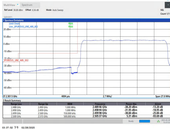
Band41_15MHz_QPSK_39765_75RB#0
