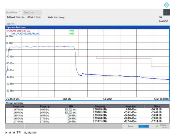
Band41_20MHz_QPSK_41490_100RB#0
