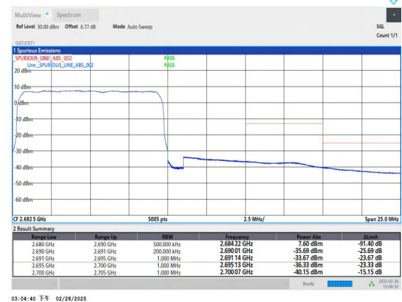
Band41_10MHz_QPSK_41540_50RB#0
