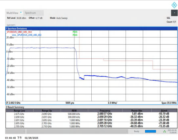
Band41_15MHz_QPSK_41515_75RB#0
