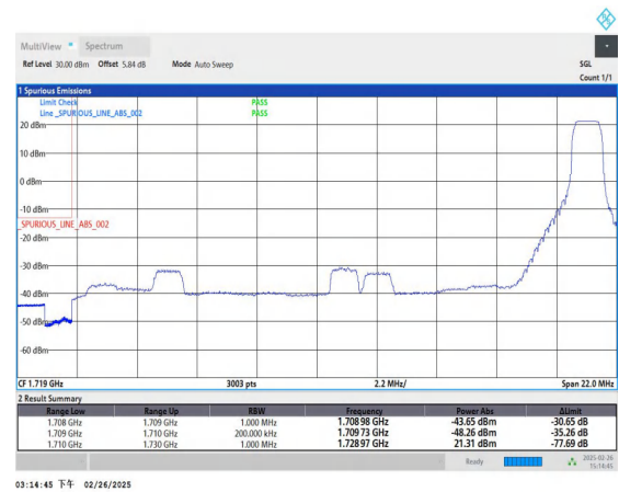
Band66_20MHz_QPSK_132072_1RB#99
