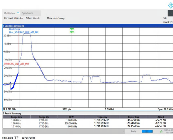
Band66_20MHz_QPSK_132072_1RB#0
