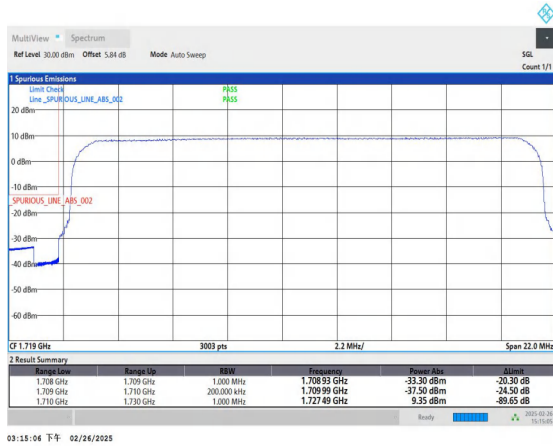
Band66_20MHz_QPSK_132072_100RB#0
