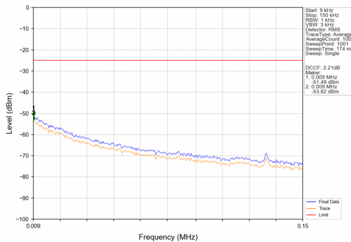
Band41_20MHz_QPSK_LCH_2565MHz_RB_1_0_NTNV
