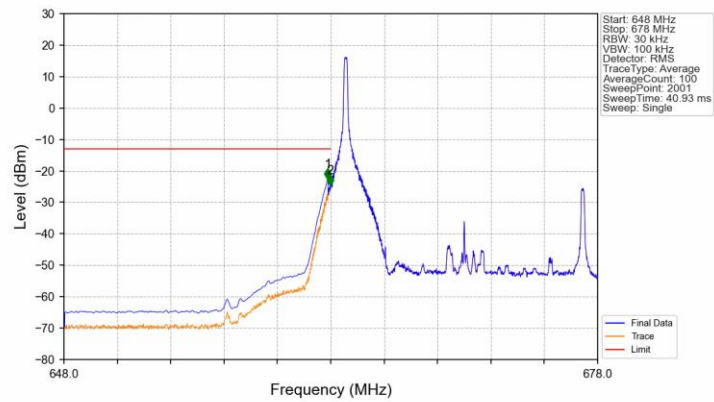
Band71_15MHz_QPSK_LCH_670.5MHz_RB_1_0_NTNV
