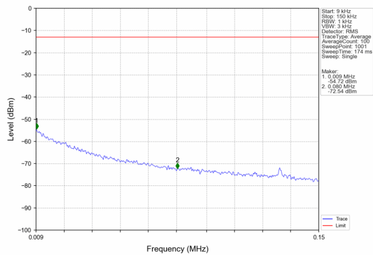
Band71_15MHz_QPSK_LCH_670.5MHz_RB_1_0_NTNV
