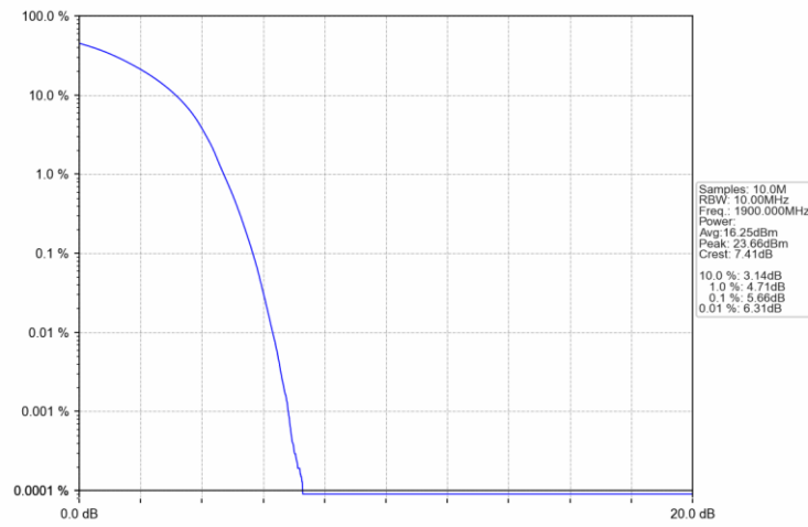
Band2_20MHz_QPSK_HCH_1900MHz_RB_100_0_NTNV
