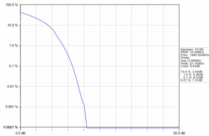
Band2_20MHz_16QAM_LCH_1860MHz_RB_100_0_NTNV
