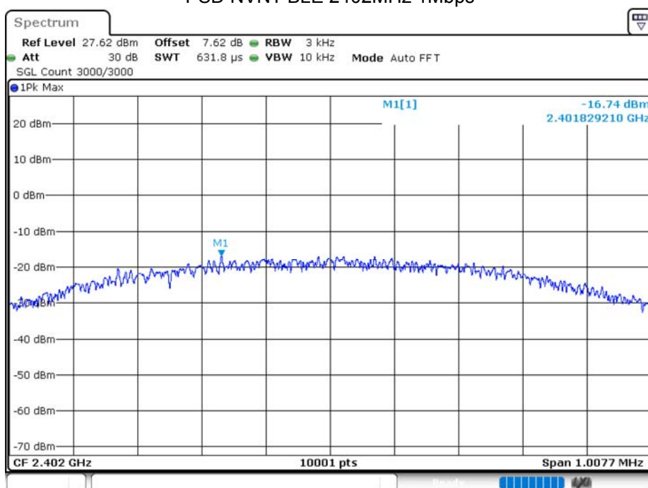
PSD NVNT BLE 2402MHz 1Mbps
