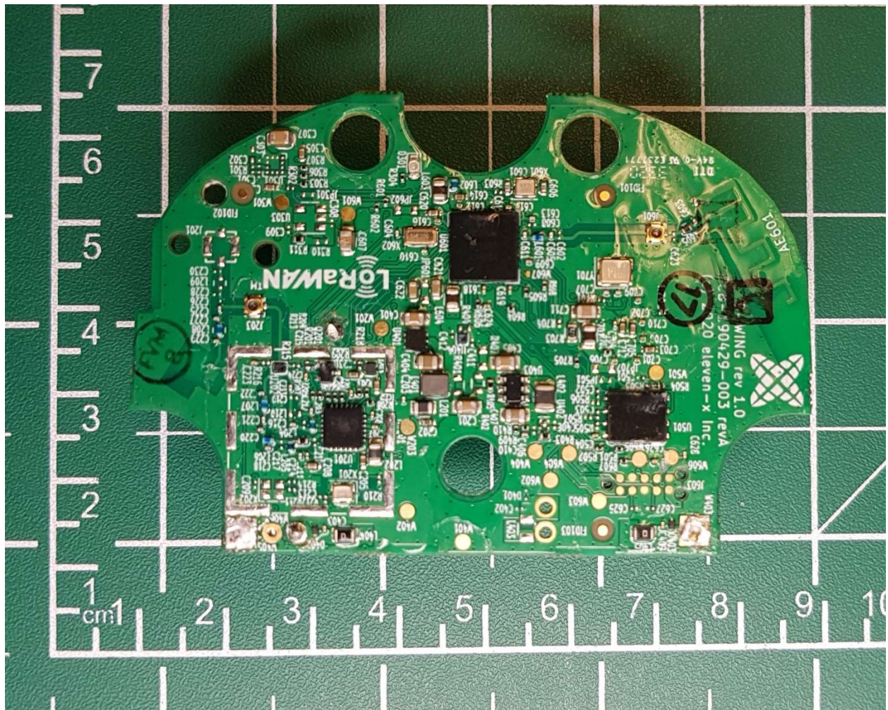
PCB bottom
