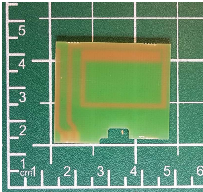
LoRa antenna PCB bottom
