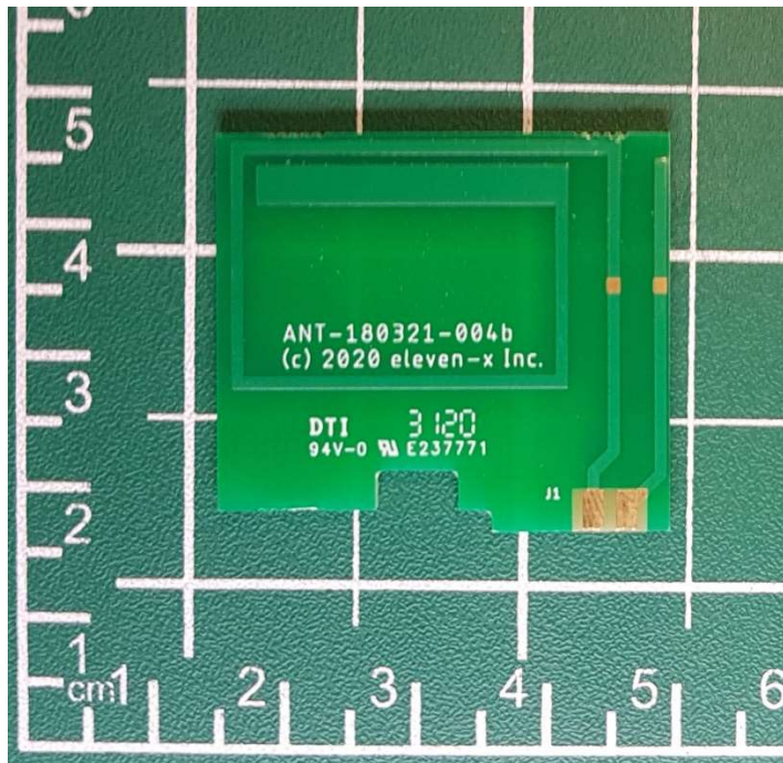
LoRa antenna PCB top
