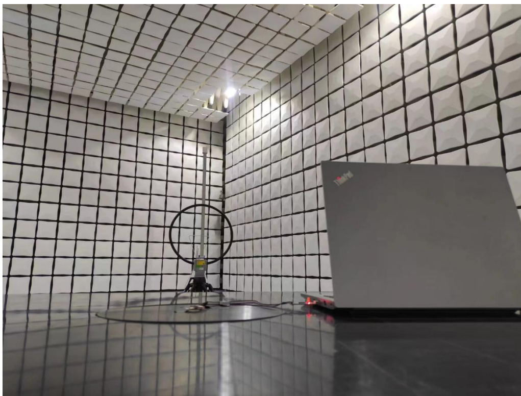
9KHz~30MHz
