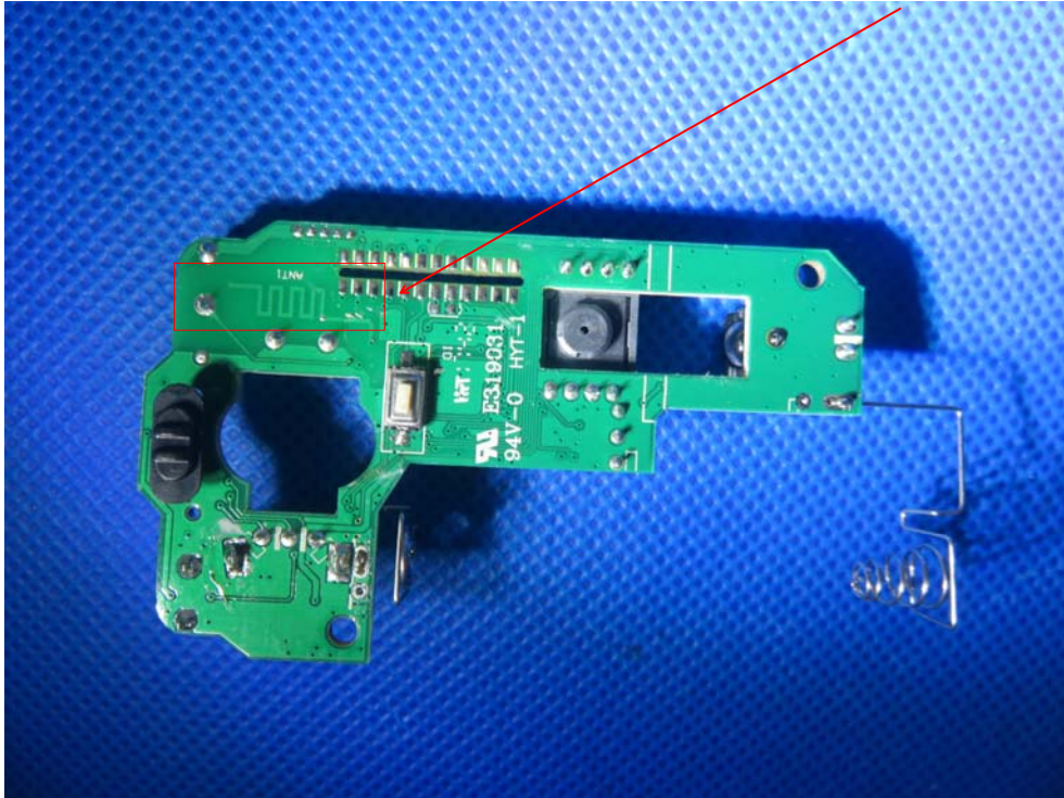
2.4GHz Antenna
