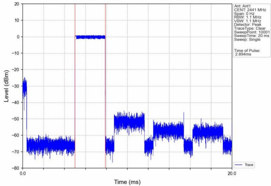
Pi/4DQPSK_2DH5_HOPP_Ant1_NTNV
