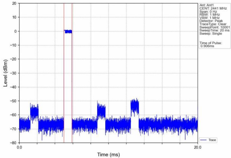
8DPSK_3DH5_HOPP_Ant1_NTNV
