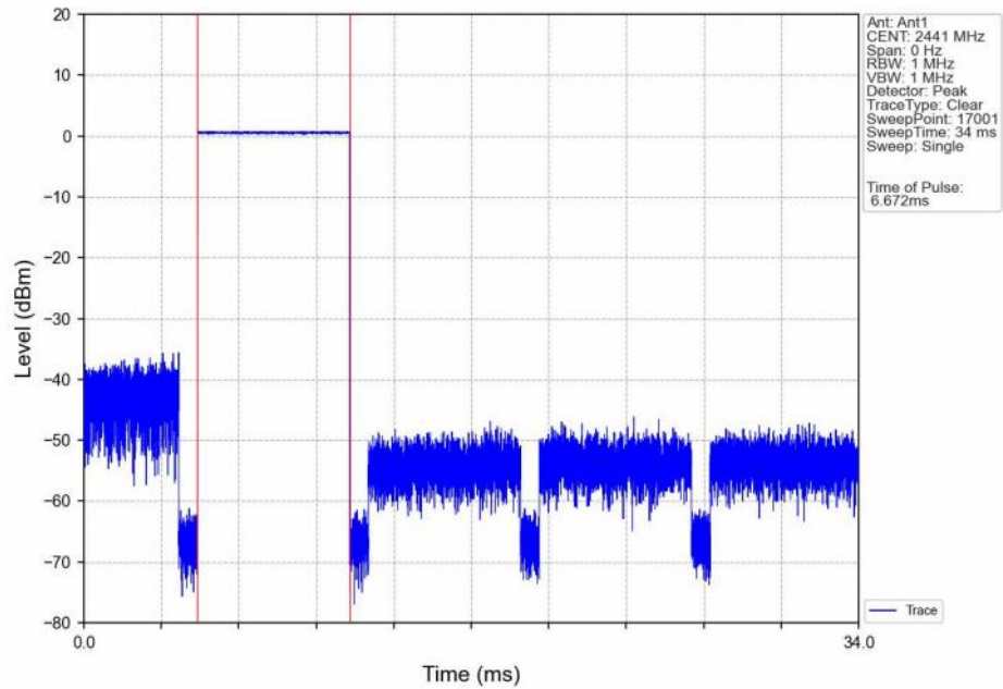
8DPSK_3DH1_HOPP_Ant1_NTNV
