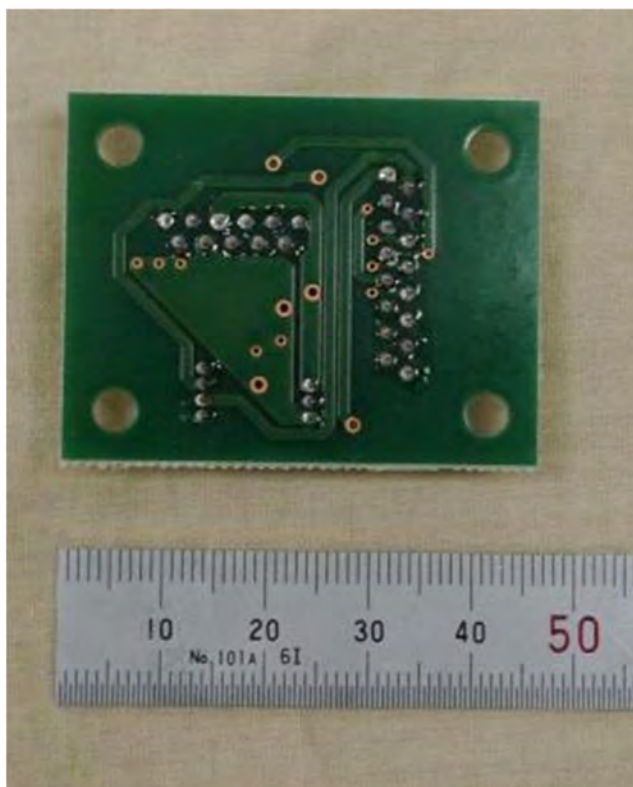
(d) Main Transfer junction board A – Bottom side
