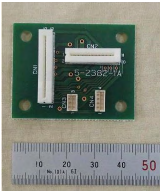
(d) Main Transfer junction board A – Top side
