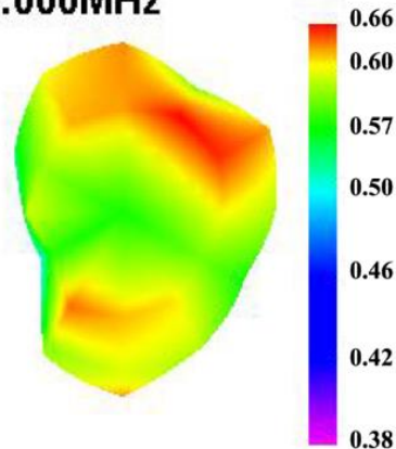
2500.000MHz
