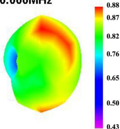
2400.000MHz
