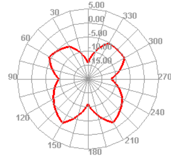
2400.000MHz E2
