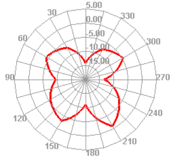
2400.000MHz E1
