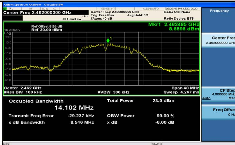
6dB Bandwidth_11B_2462_Ant1
