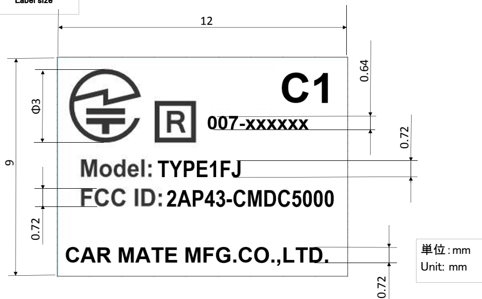
ラベル寸法 Label size
