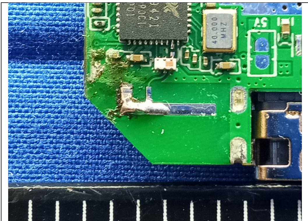
Antenna
