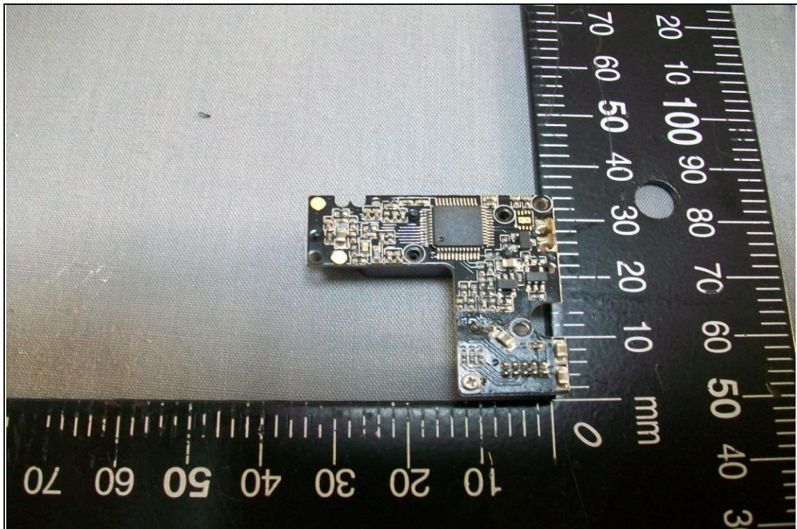
< PCB6-F >
