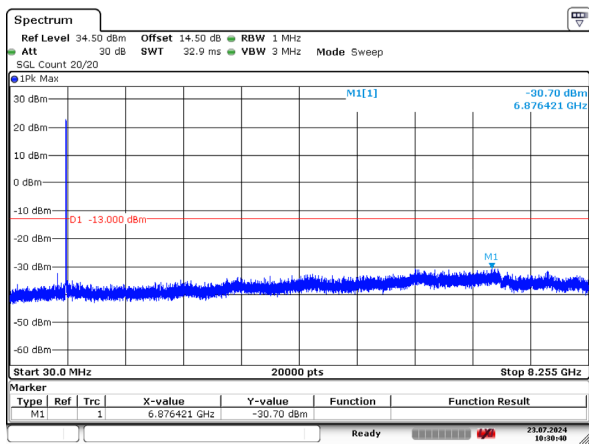
2_3MHz_Low_QPSK_15@0
