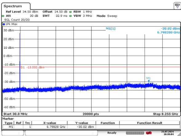
2_3MHz_Low_QPSK_1@0
