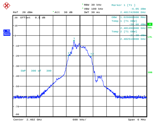
Low 1.020MHz
