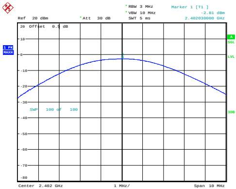
Low -2.81dBm
