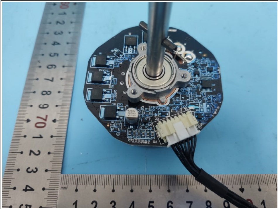
Fig. 51 Motor
