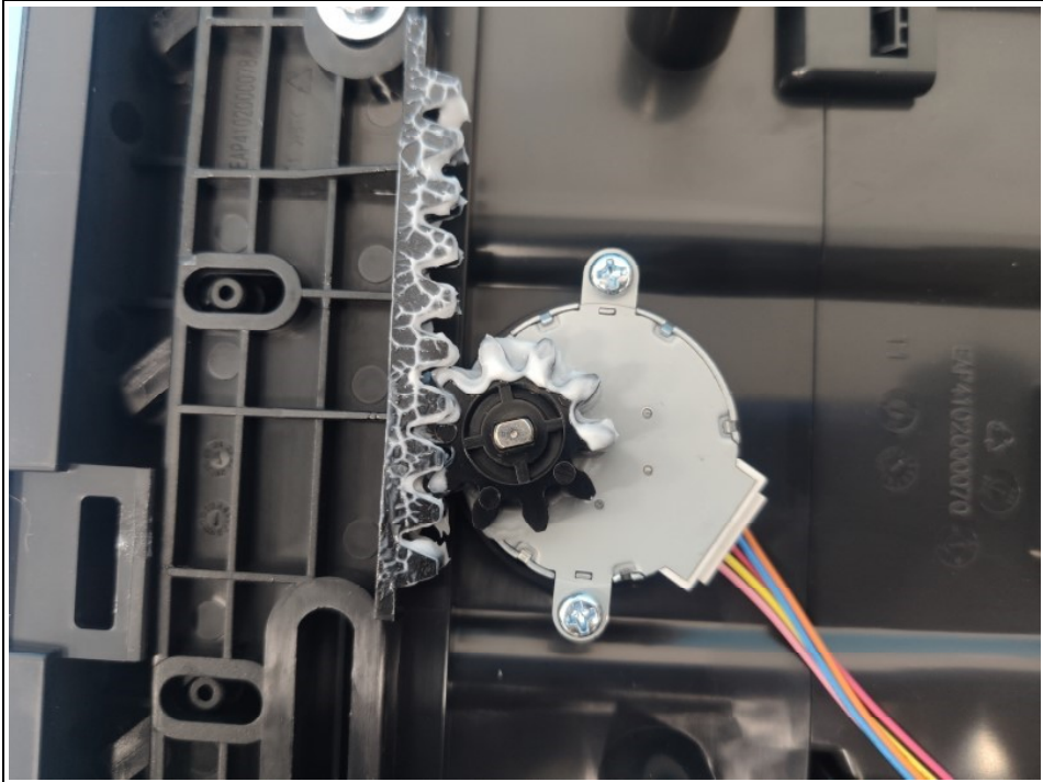
Fig. 40 Stepper motor
