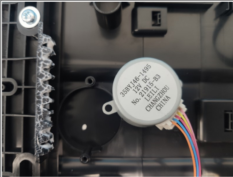
Fig. 41 Stepper motor
