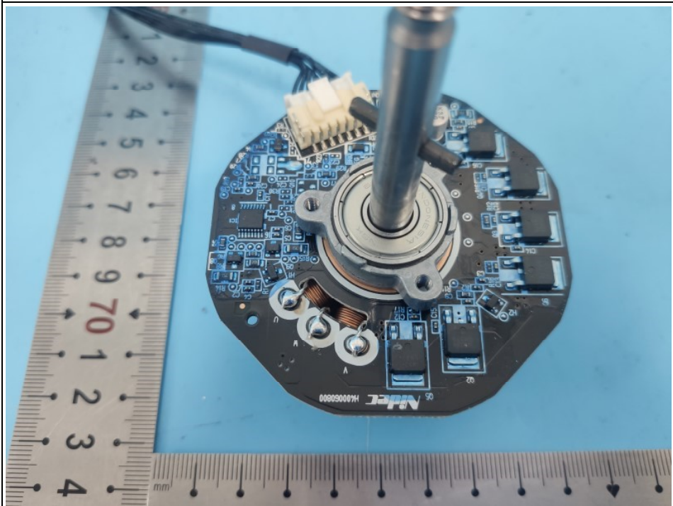
Fig. 50 Motor
