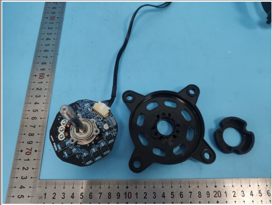
Fig. 48 Motor
