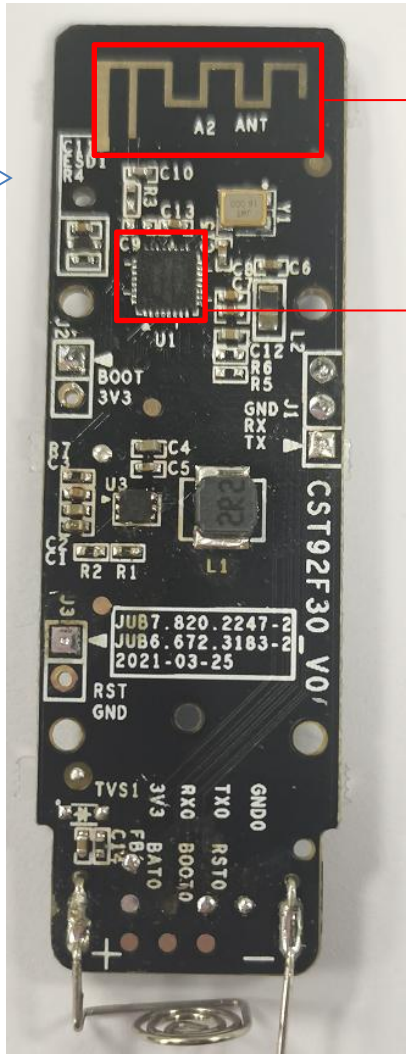
PCBA- BOTTOM
