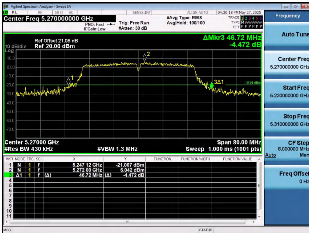
11N40SISO-Ant1-5270
