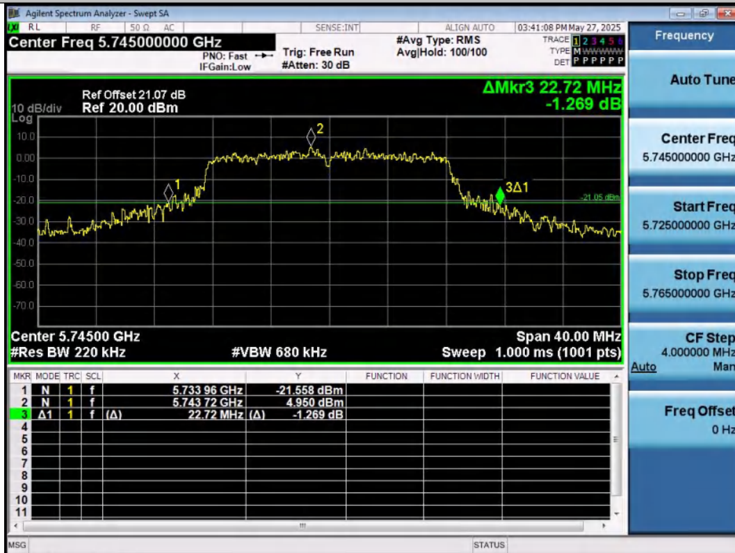
11A-Ant1-5745
