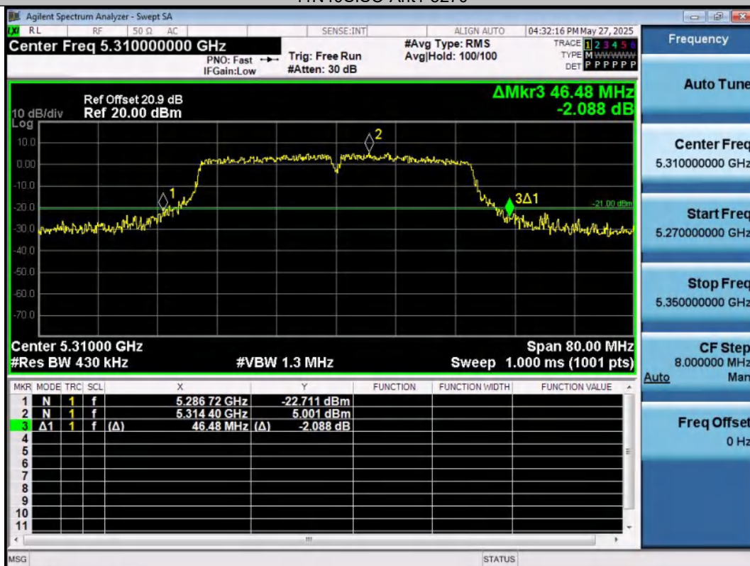
11N40SISO-Ant1-5310
