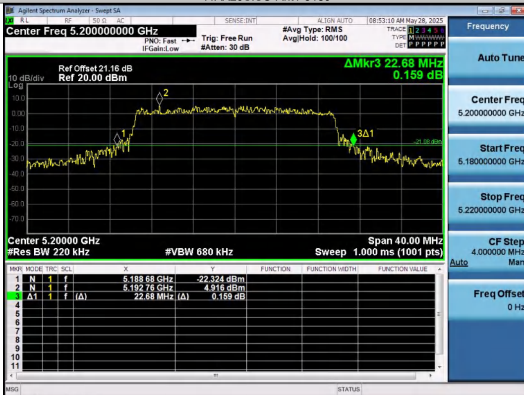
11AX20SISO-Ant1-5200
