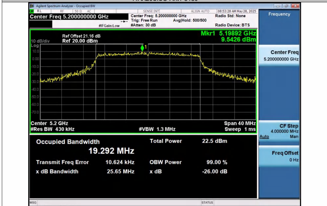
11AX20SISO-Ant1-5200
