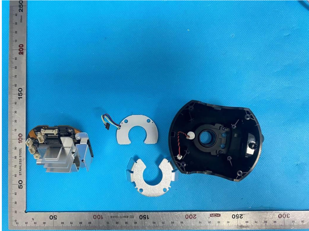
ANTANNA
