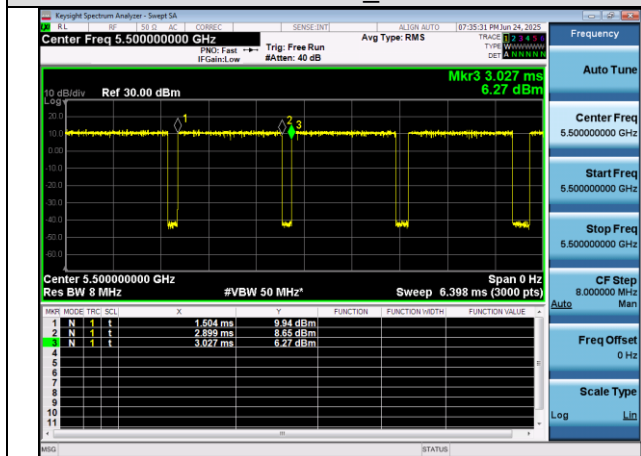
IEEE 802.11n-HT40_U-NII 2C
