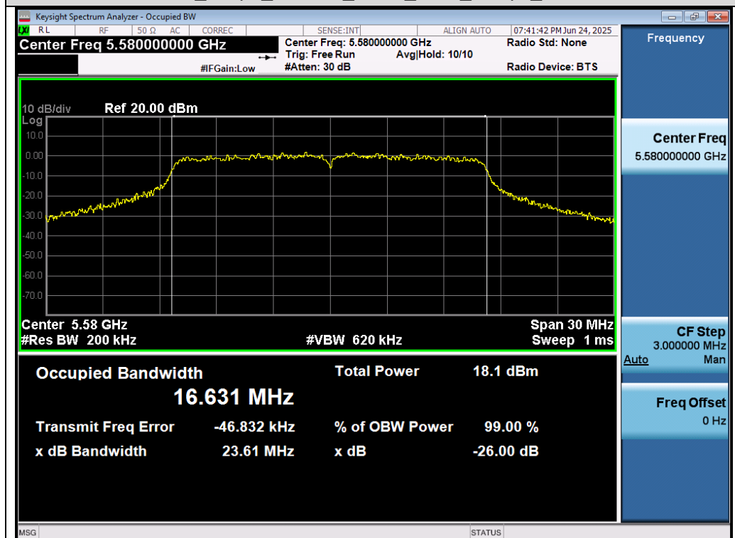
Test_Graph_802.11a_ANT1_5580_6Mbps_OBW
