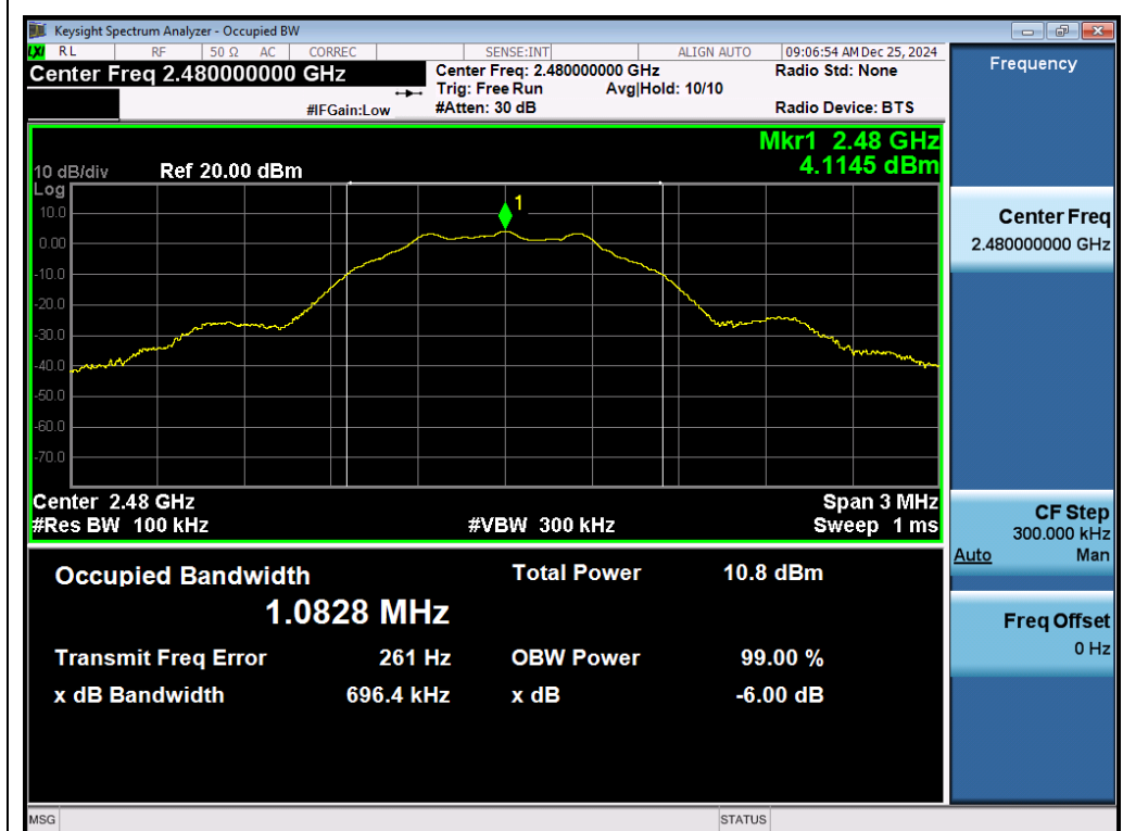
Test_Graph_LE1M_ANT1_2480_1Mbps_DTSSBW
