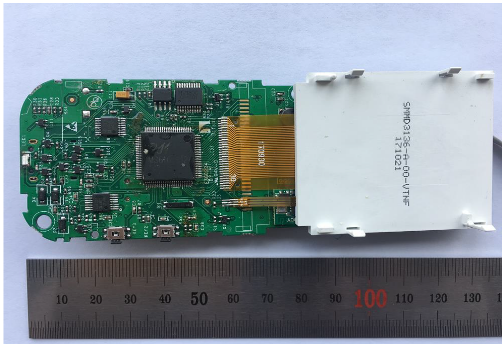
(4) EUT Photo
