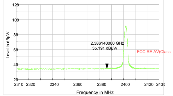
BLE Channel 0 Average
