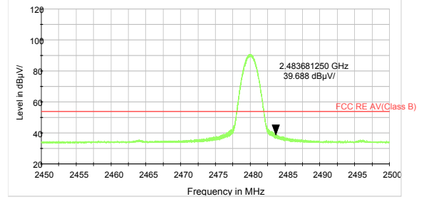
BLE Channel 39 Average
