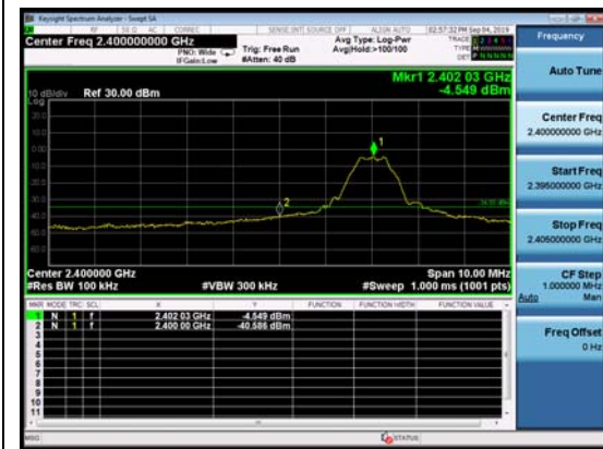
BLE V4.2, Channel No.: 0
