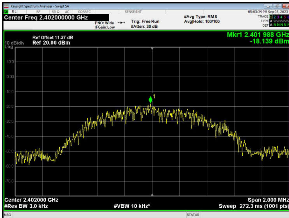
PSD BLE (1M) 2402MHz
