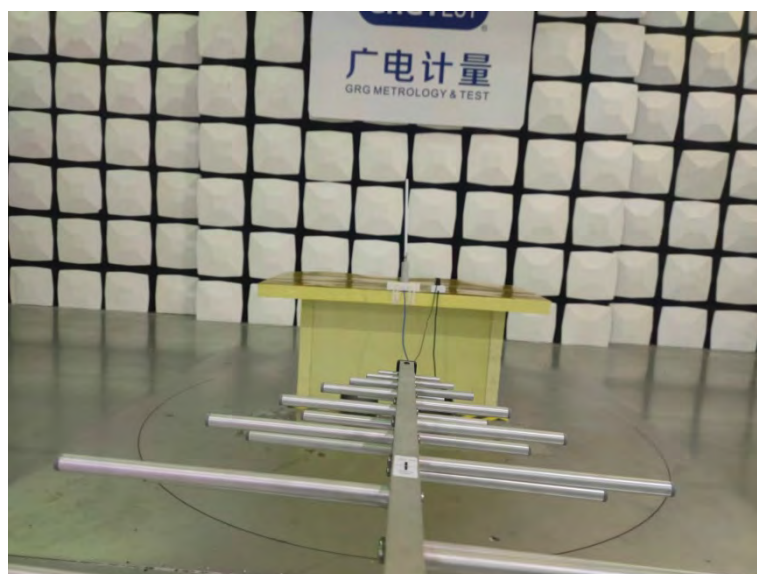
30MHz ~ 1GHz
