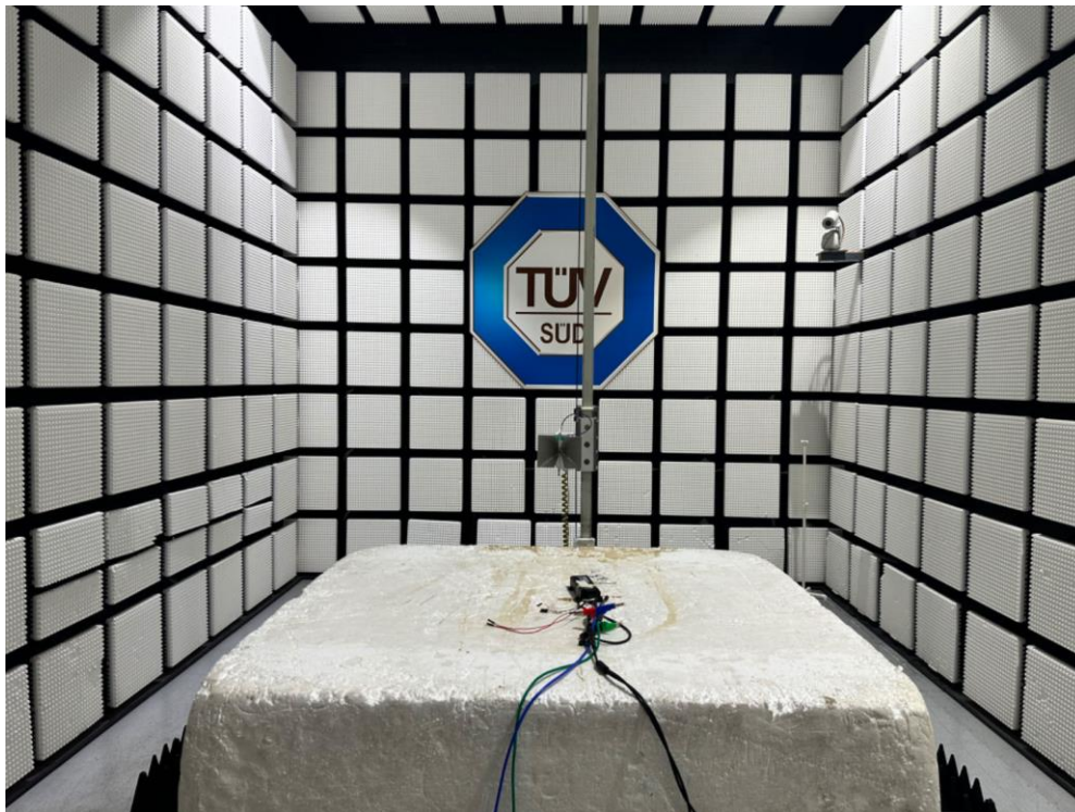
1GHz ~ 18GHz
