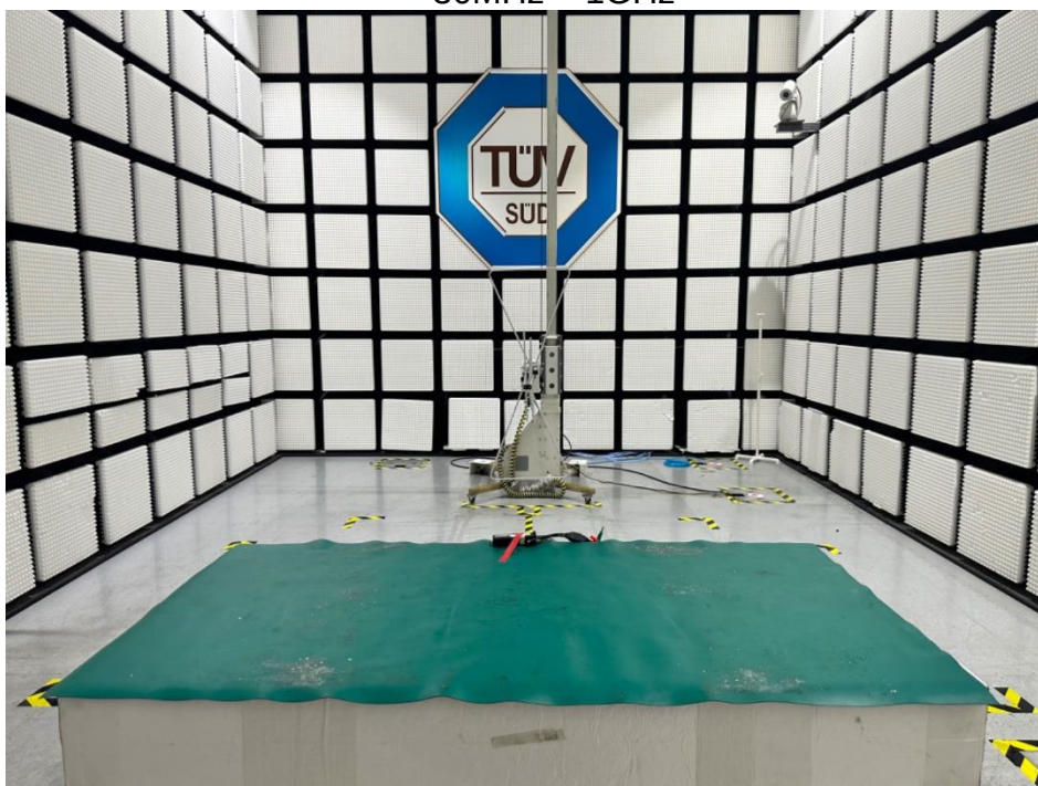
30MHz ~ 1GHz
