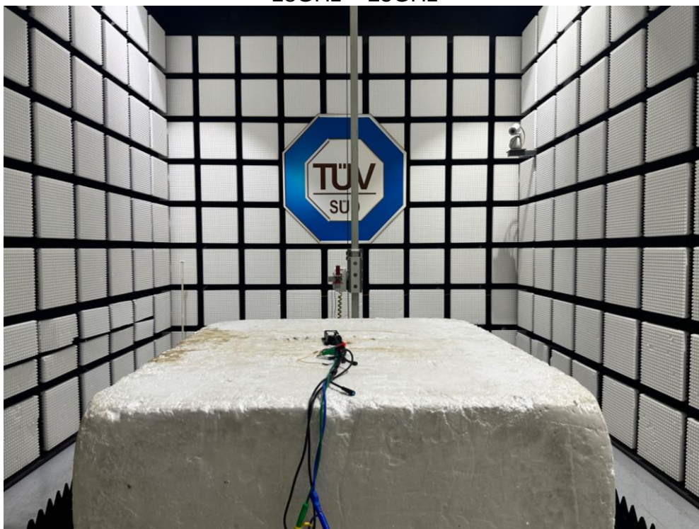
18GHz ~ 25GHz
