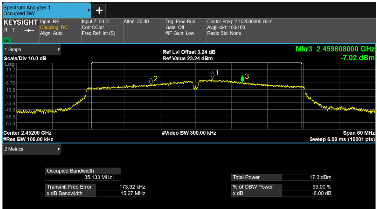
-6dB Bandwidth NVNT n40 2452MHz Ant1
