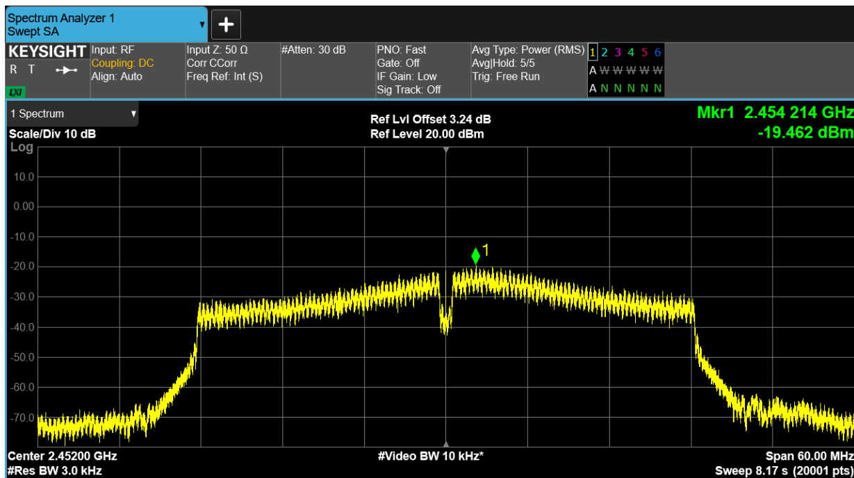
PSD NVNT n40 2452MHz Ant1
