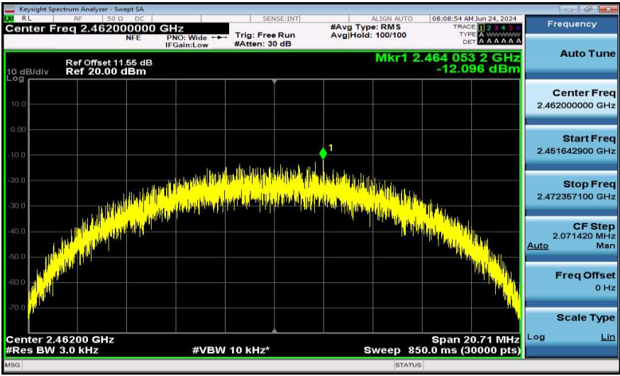
11B-Ant2-2462-PASS
